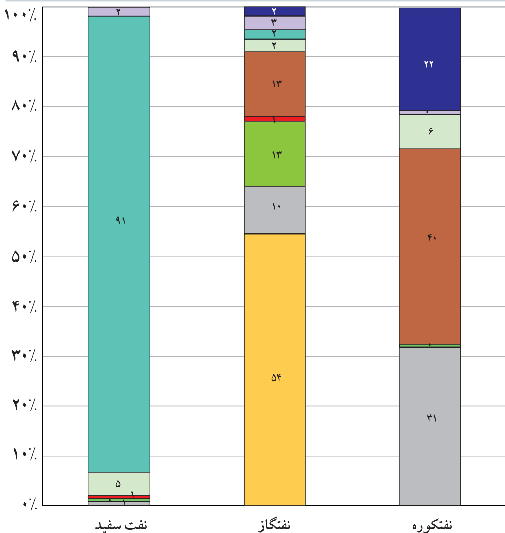
نمودار درصد مصرف نفت سفید نفتگاز و نفتکوره در بخش های مختلف مصرف در سال ۱۳۸۷
